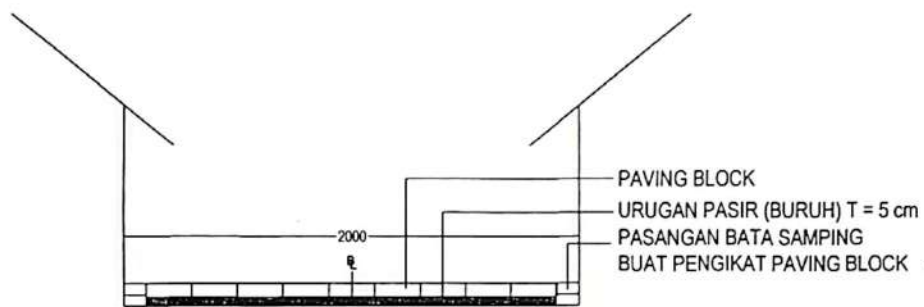
STA. 0+000 - STA. 0+012 STA. 0+000 - STA. 0+020 DETAIL KONSTRUKSI JALAN
